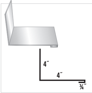
#37 SS Sidewall
