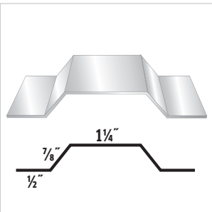
#82 Hat Channel
